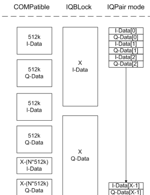
Fig. 1-1: I/Q data formats
